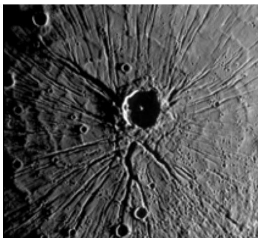
Меркурий
