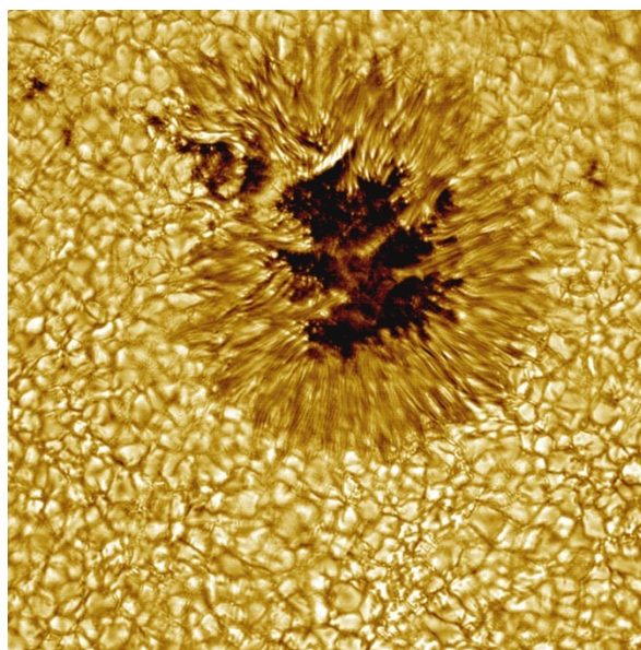
Солнце
