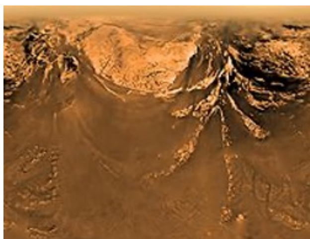
Титан
