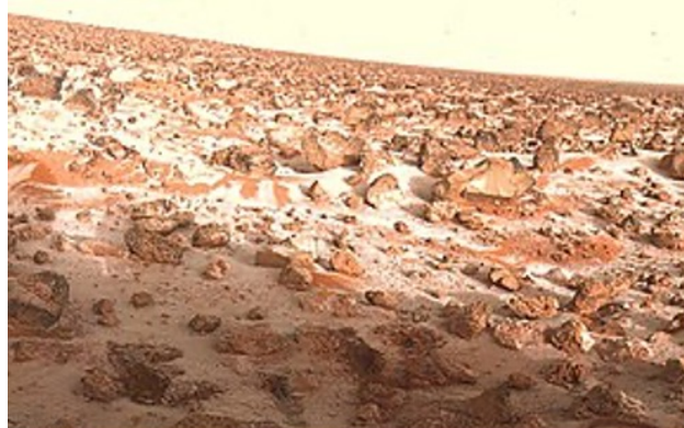
Марс
